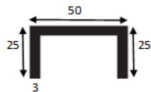
PROFIL U 25X50X25X3
