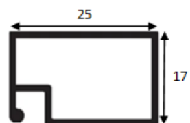
PROFIL PLASA 17X25
