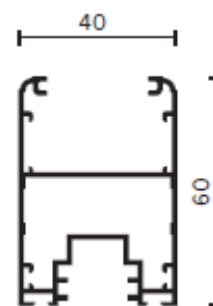
ELVIAL EL8111
