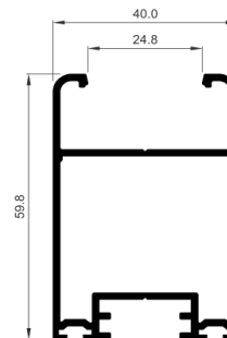
CORTIZO COR-2445
