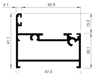
CORTIZO COR-2422
