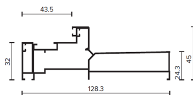
ELVIAL EL8107
