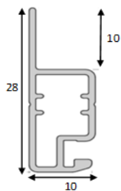
PROFIL PLASA 10X28
