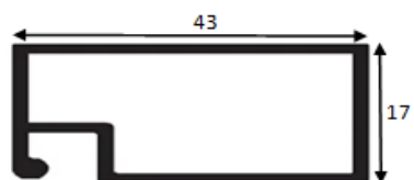
PROFIL PLASA 17X43
