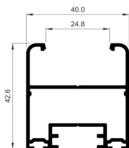
CORTIZO COR-2425
