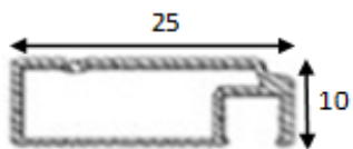
PROFIL PLASA BELCO 10X25
