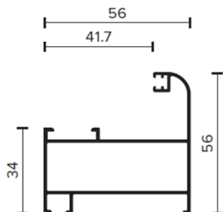
ELVIAL EL2132
