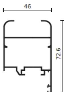
ELVIAL EL2110
