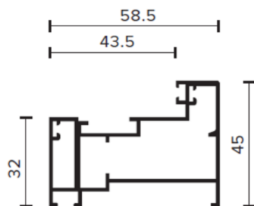
ELVIAL EL8102
