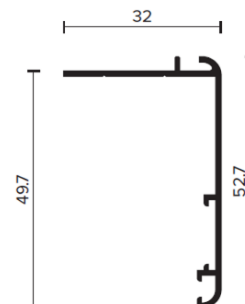
ELVIAL EL2096
